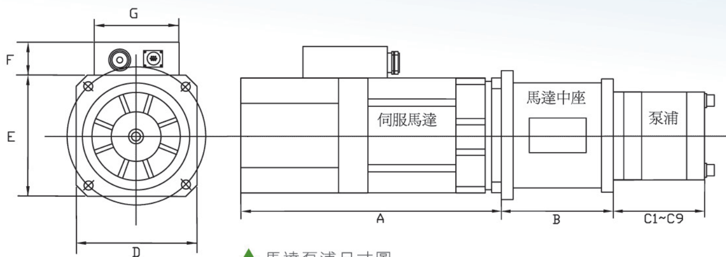
▲ 馬達泵浦尺寸圖
